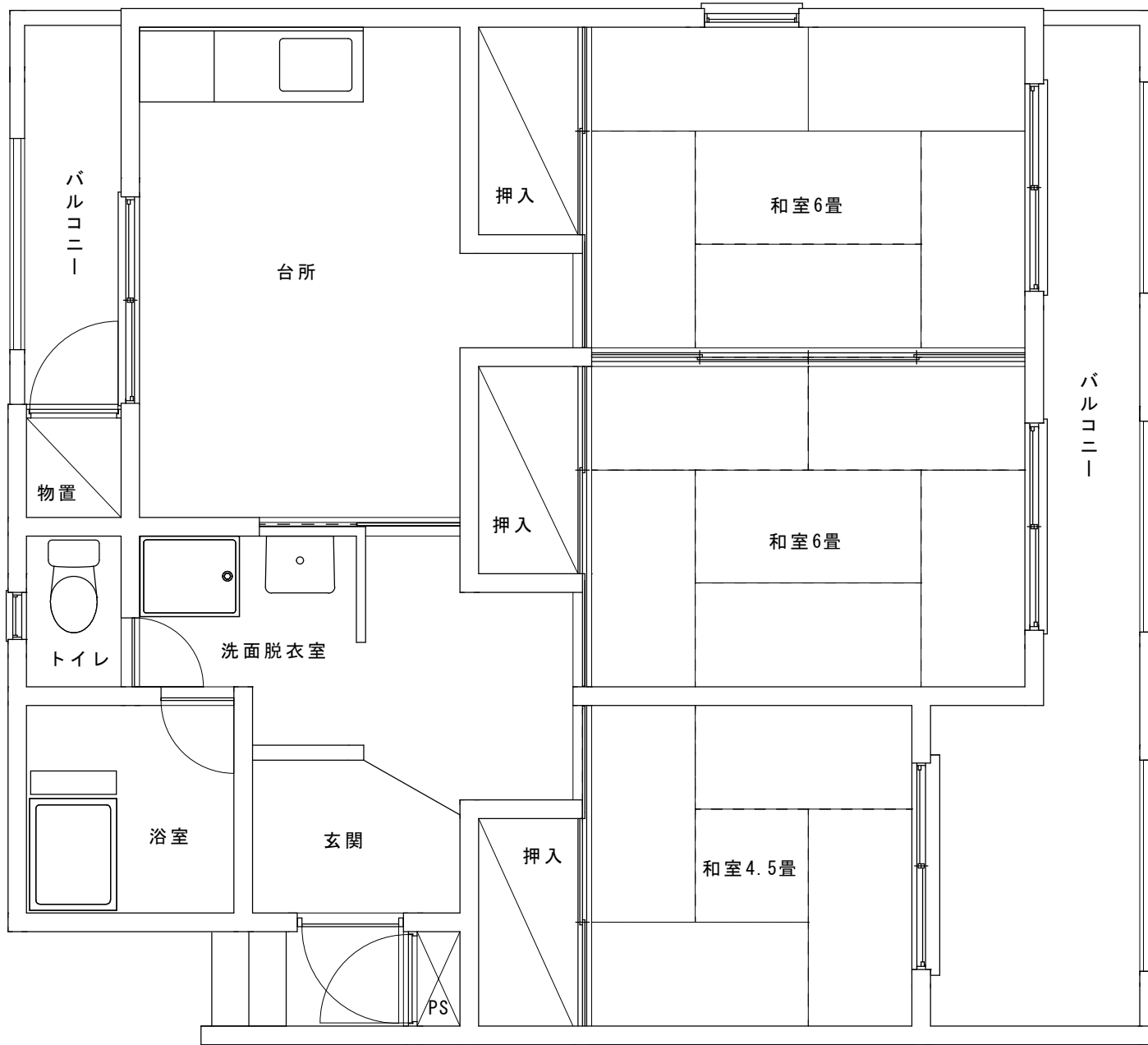
思勝団地 村営住宅3号棟 102
